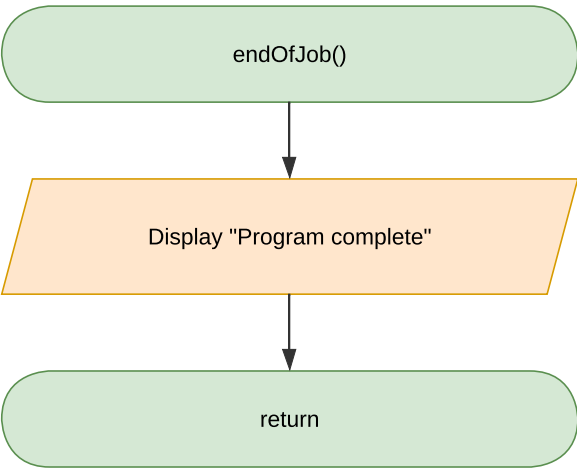
endOfJob() Module
