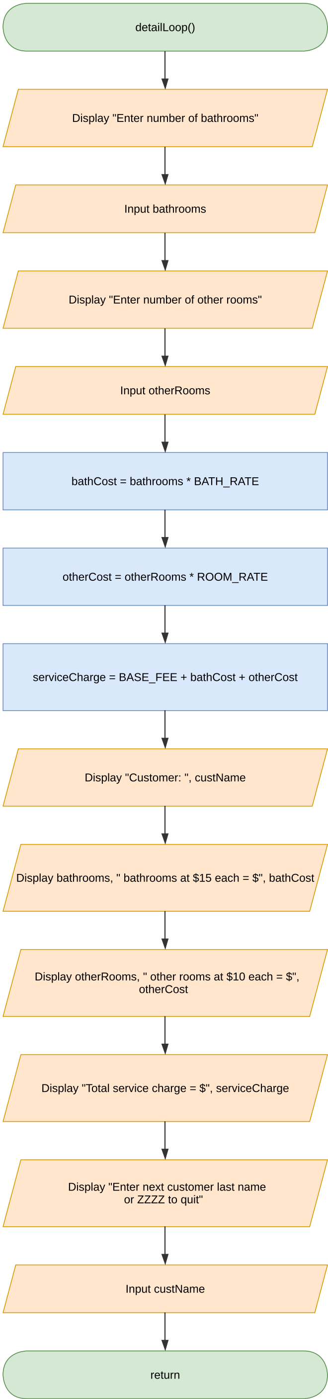
detailLoop() Module
